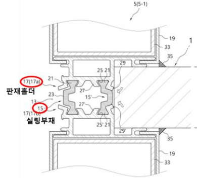
<창호시스템 세로바의 단면도>
