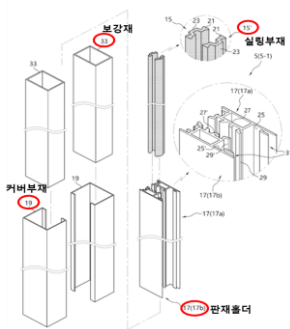
<창호시스템 분해 사시도>
